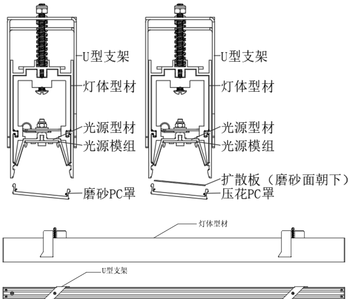
灯具顶面结构
